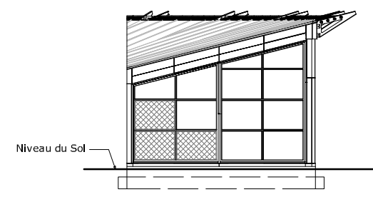
Vue C
