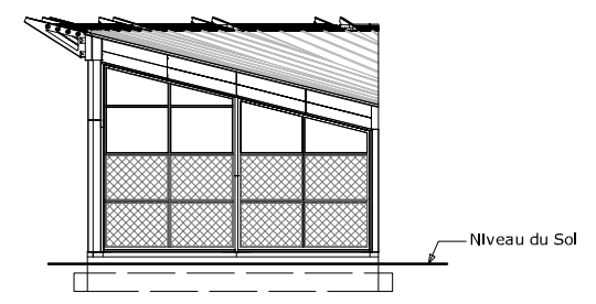
Vue D
