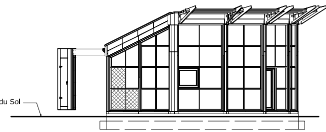
Vue E
