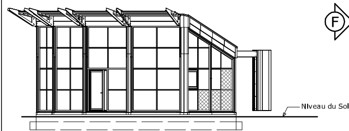
Vue F
