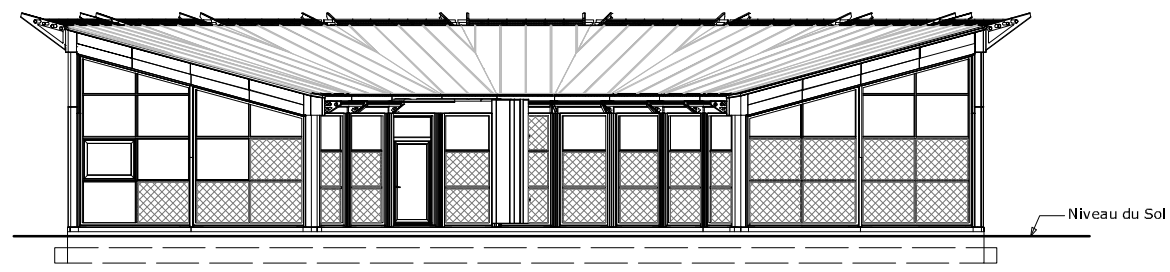
Vue A
