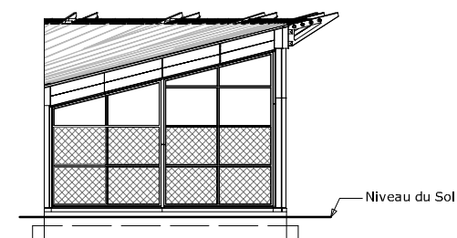
Vue C
